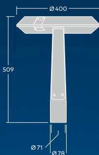
Ø 71 mm pour emmanchement Ø 60 mm
