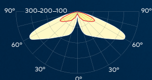
Optique de révolution symétrique (RS)
