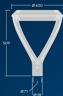
Ø 71 mm pour emmanchement Ø 60 mm
