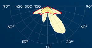
Optique asymétrique pour rue (STR-A)
